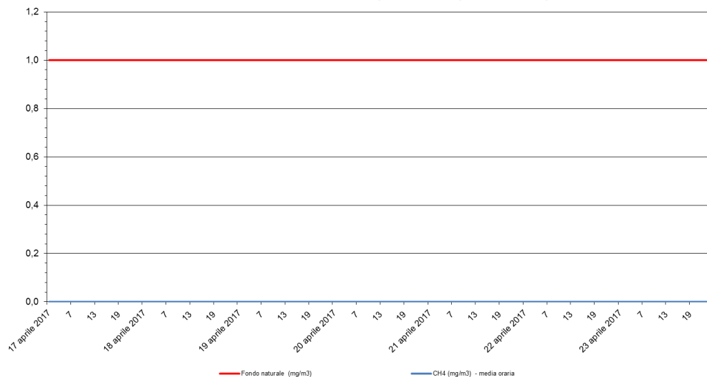
Metano - CH 4 Stazione di rilevamento di via B. Cairoli, periodo: 17 apr 2017 - 23 apr 2017
