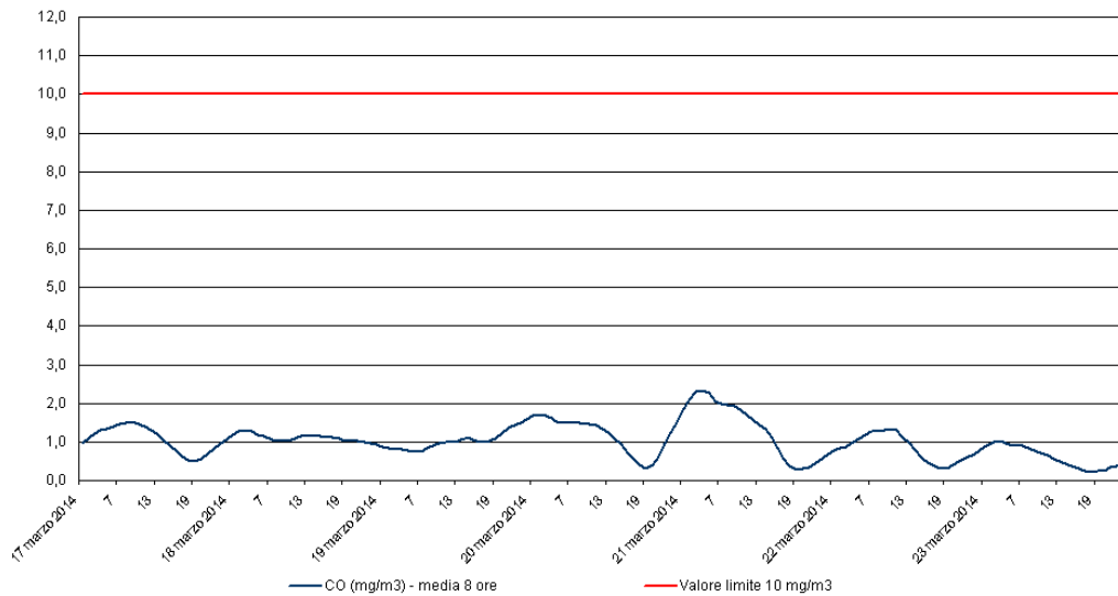
Monossido di Carbonio - CO Stazione di rilevamento di Sambruson, periodo: 17 mar 2014 - 23 mar 2014
