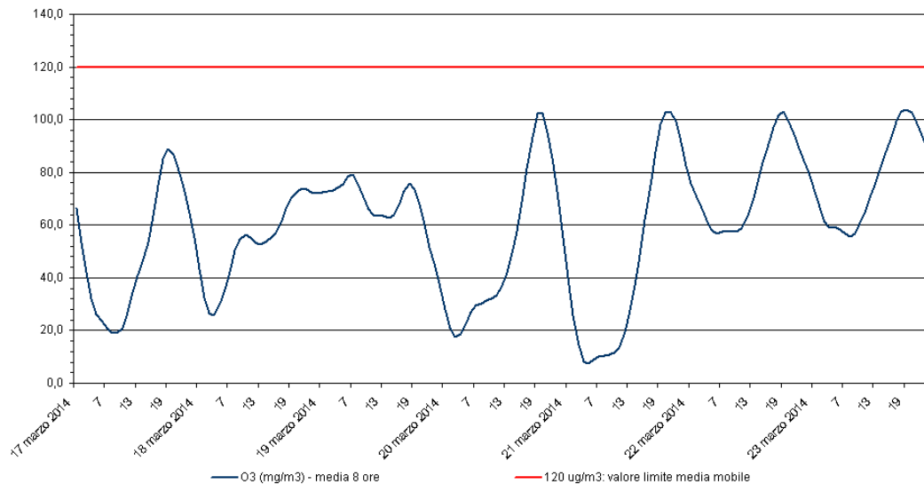
Ozono - O 3 Stazione di rilevamento di Sambruson, periodo: 17 mar 2014 - 23 mar 2014
