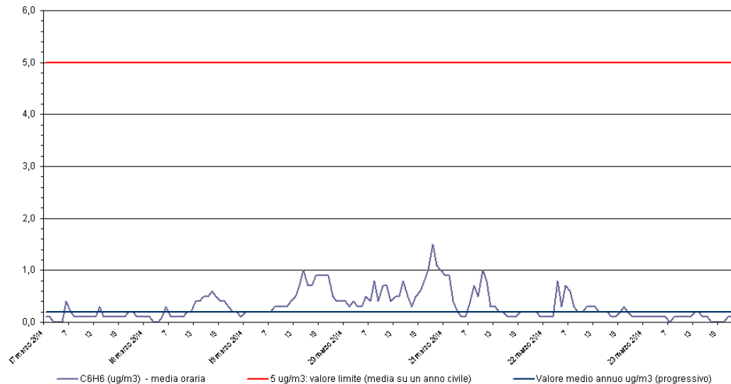
Benzene - C 6 H 6 Stazione di rilevamento di Sambruson, periodo: 17 mar 2014 - 23 mar 2014
