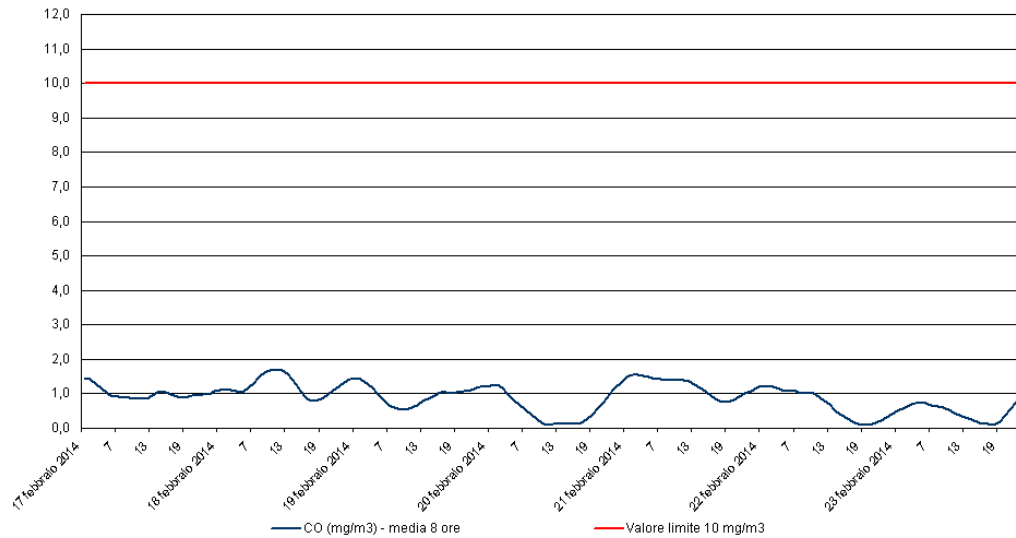
Monossido di Carbonio - CO Stazione di rilevamento di Sambruson, periodo: 17 feb 2014 - 23 feb 2014
