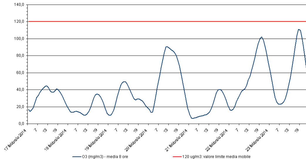
Ozono - O 3 Stazione di rilevamento di Sambruson, periodo: 17 feb 2014 - 23 feb 2014
