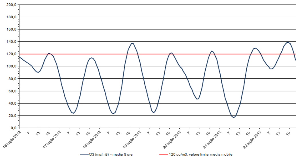
Ozono - O3 Stazione di rilevamento di via B. Cairoli, periodo: 16 lug 2012- 22 lug 2012
