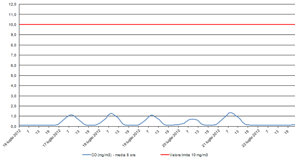
Monossido di Carbonio - CO Stazione di rilevamento di via B. Cairoli, periodo: 16 lug 2012- 22 lug 2012
