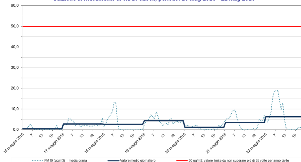
PM10 Stazione di rilevamento di via B. Cairoli, periodo: 16 mag 2016 - 22 mag 2016
