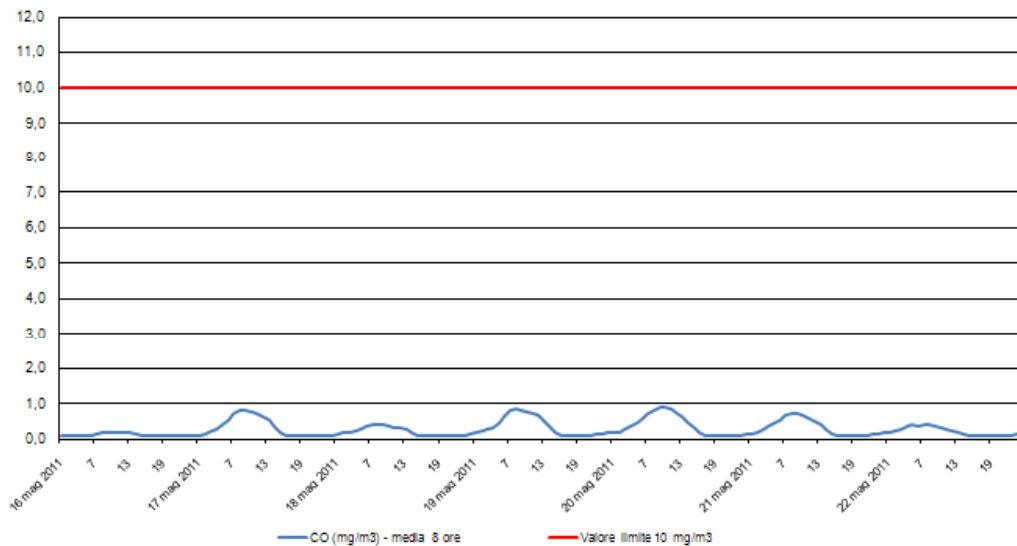
Monossido di Carbonio - CO Stazione di rilevamento di via B. Cairoli, periodo: 16 mag 2011 - 22 mag 2011
