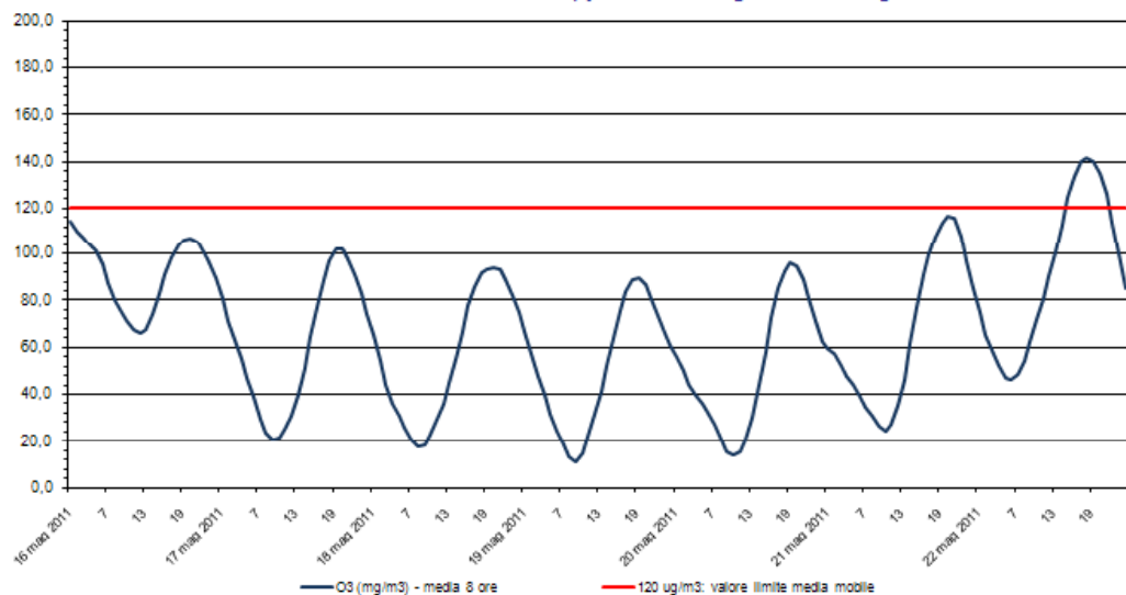
Ozono - O 3 Stazione di rilevamento di via B. Cairoli, periodo: 16 mag 2011 - 22 mag 2011
