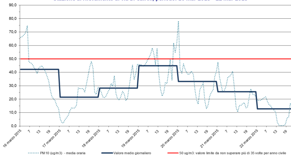
PM10 Stazione di rilevamento di via B. Cairoli, periodo: 16 mar 2015 - 22 mar 2015
