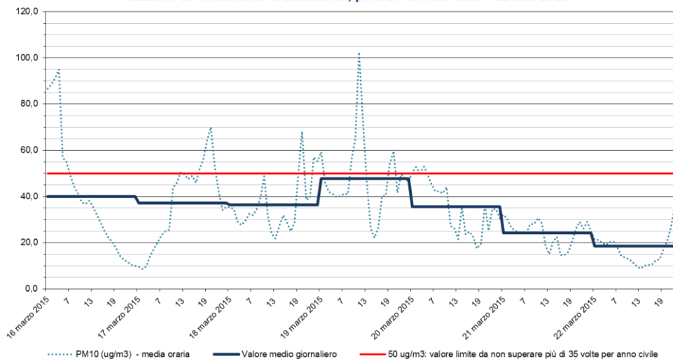
PM10 Stazione di rilevamento di Sambruson, periodo: 16 mar 2015 - 22 mar 2015
