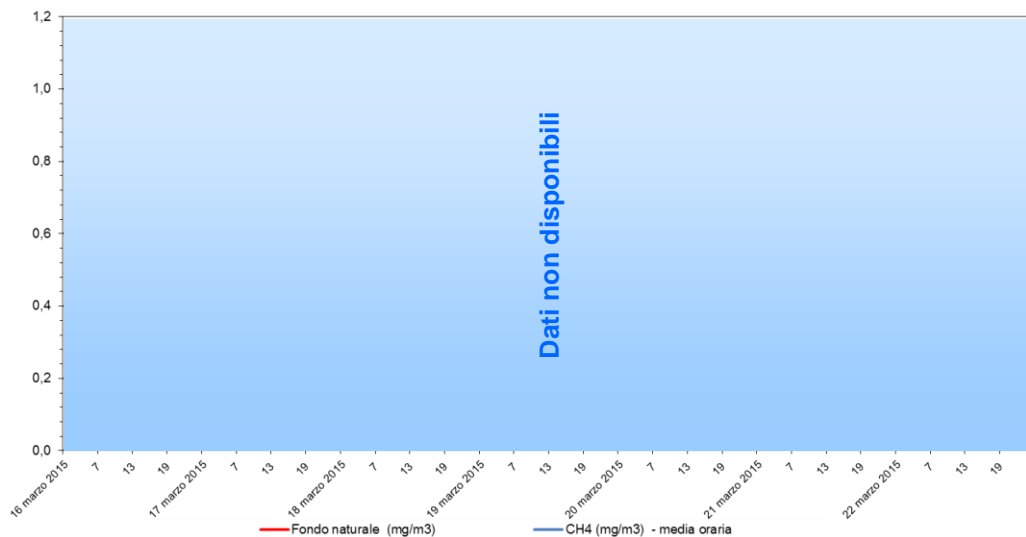
Metano - CH 4 Stazione di rilevamento di Sambruson, periodo: 16 mar 2015 - 22 mar 2015
