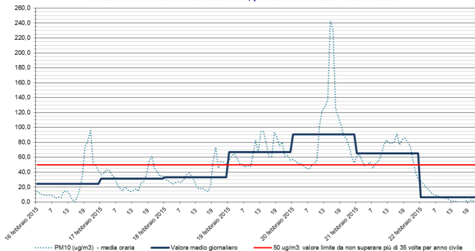
PM10 Stazione di rilevamento di Sambruson, periodo: 16 feb 2015 - 22 feb 2015
