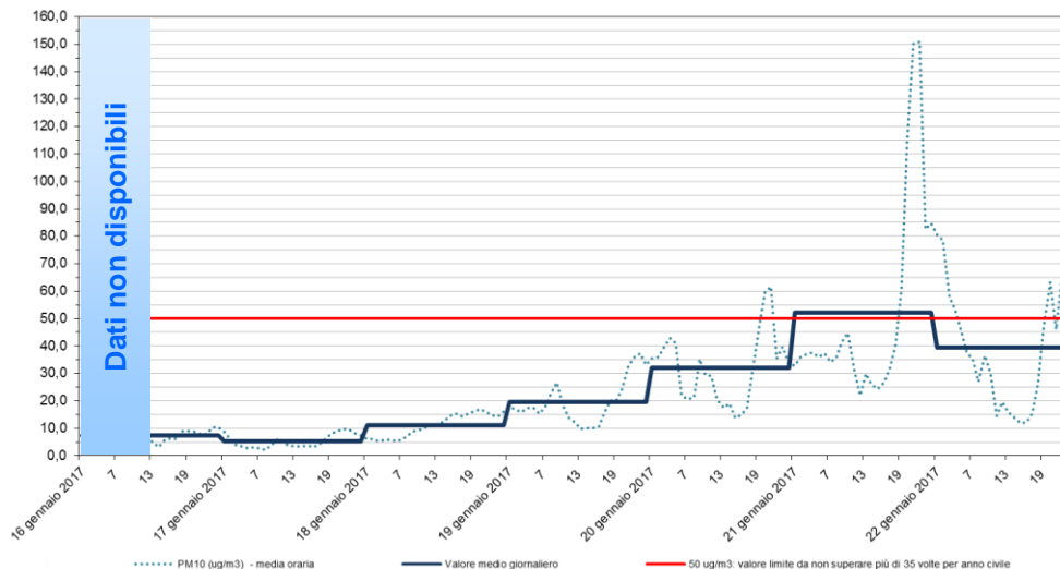
PM10 Stazione di rilevamento di via B. Cairoli, periodo: 16 gen 2017 - 22 gen 2017
