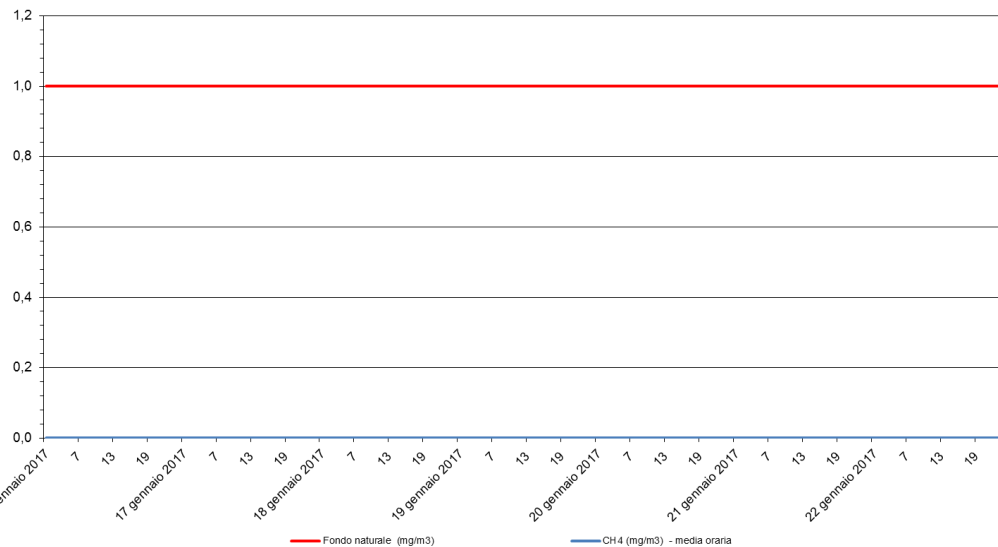
Metano - CH 4 Stazione di rilevamento di via B. Cairoli, periodo: 16 gen 2017 - 22 gen 2017
