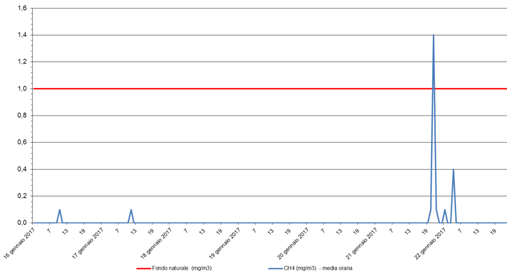
Metano - CH 4 Stazione di rilevamento di Sambruson, periodo: 16 gen 2017 - 22 gen 2017
