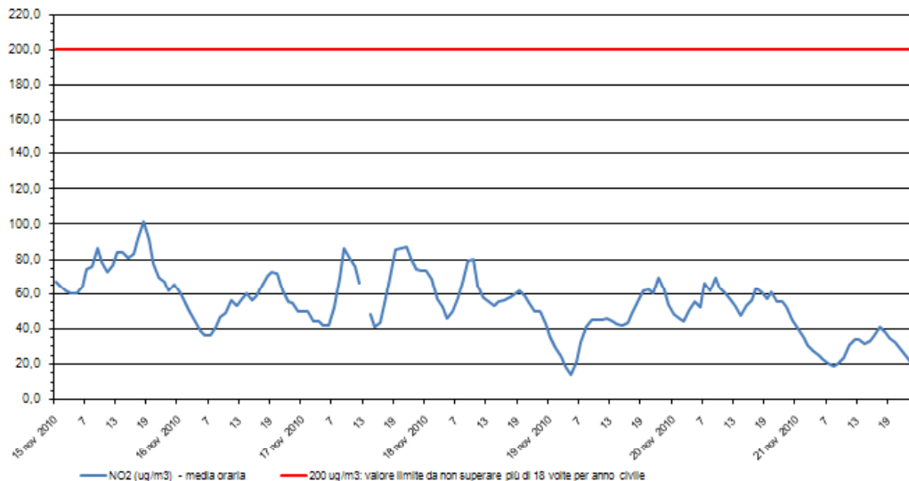
Biossido di azoto - NO 2 Stazione di rilevamento di via B. Cairoli, periodo: 15 nov 2010 - 21 nov 2010
