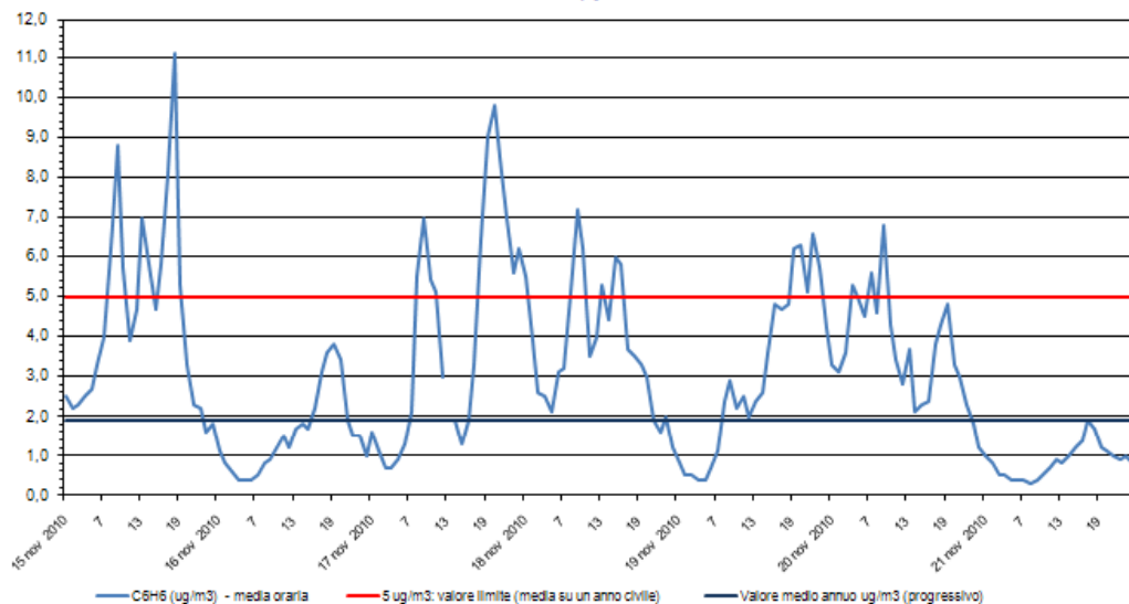
Benzene - C 6 H 6 Stazione di rilevamento di via B. Cairoli, periodo: 15 nov 2010 - 21 nov 2010
