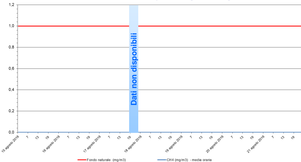
Metano - CH 4 Stazione di rilevamento di Sambruson, periodo: 15 ago 2016 - 21 ago 2016
