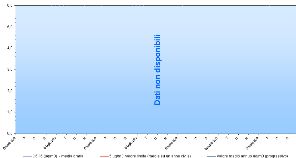
Benzene - C 6 H 6 Stazione di rilevamento di Sambruson, periodo: 15 lug 2013 - 21 lug 2013
