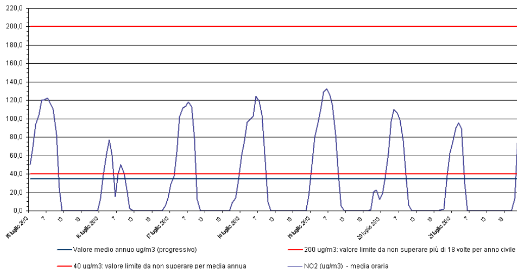
Biossido di azoto - NO 2 Stazione di rilevamento di Sambruson, periodo: 15 lug 2013 - 21 lug 2013
