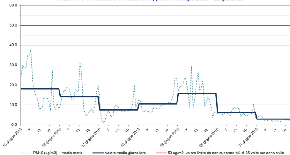
PM10 Stazione di rilevamento di Sambruson, periodo: 15 giu 2015 - 21 giu 2015
