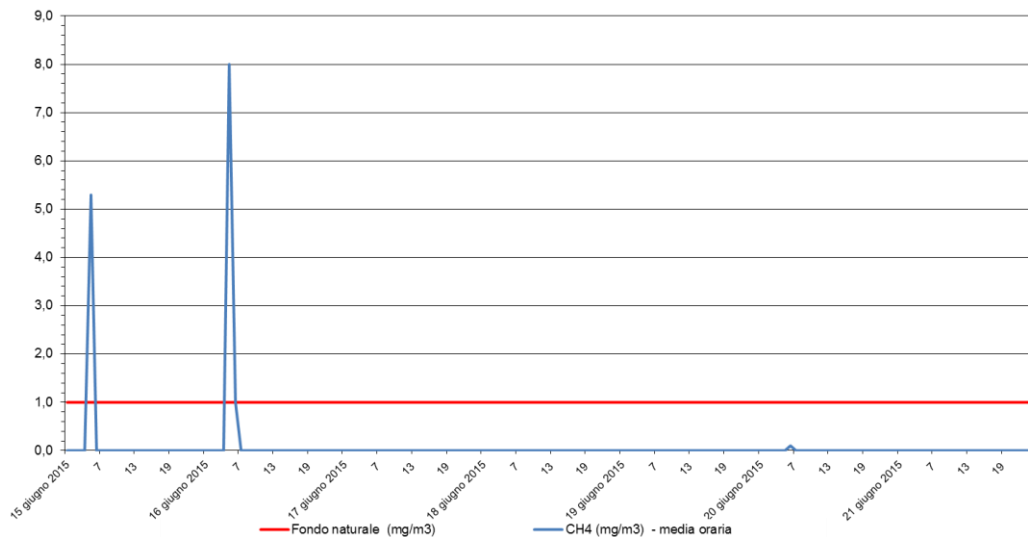
Metano - CH 4 Stazione di rilevamento di Sambruson, periodo: 15 giu 2015 - 21 giu 2015
