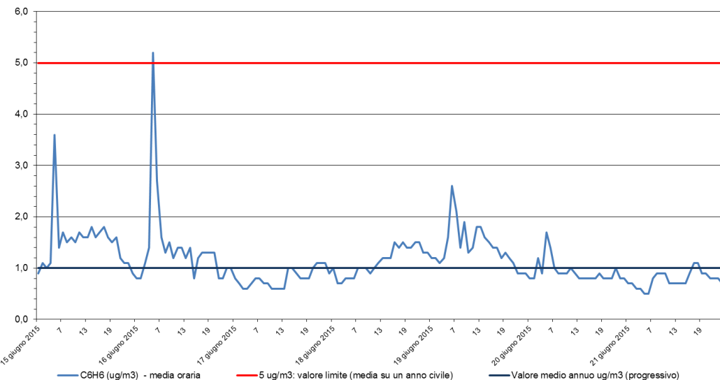
Benzene - C 6 H 6 Stazione di rilevamento di Sambruson, periodo: 15 giu 2015 - 21 giu 2015
