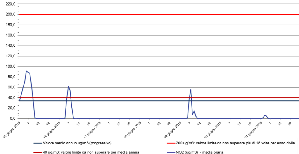
Biossido di azoto - NO 2 Stazione di rilevamento di Sambruson, periodo: 15 giu 2015 - 21 giu 2015
