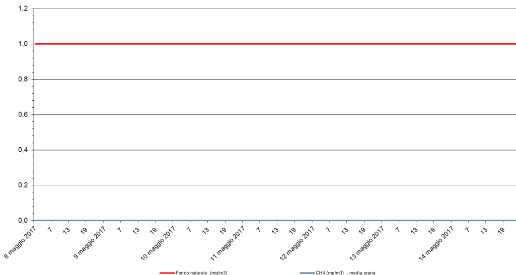
Metano - CH 4 Stazione di rilevamento di via B. Cairoli, periodo: 08 mag 2017 - 14 mag 2017
