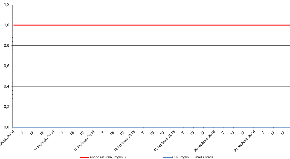
Metano - CH 4 Stazione di rilevamento di via B. Cairoli, periodo: 15 feb 2016 - 21 feb 2016
