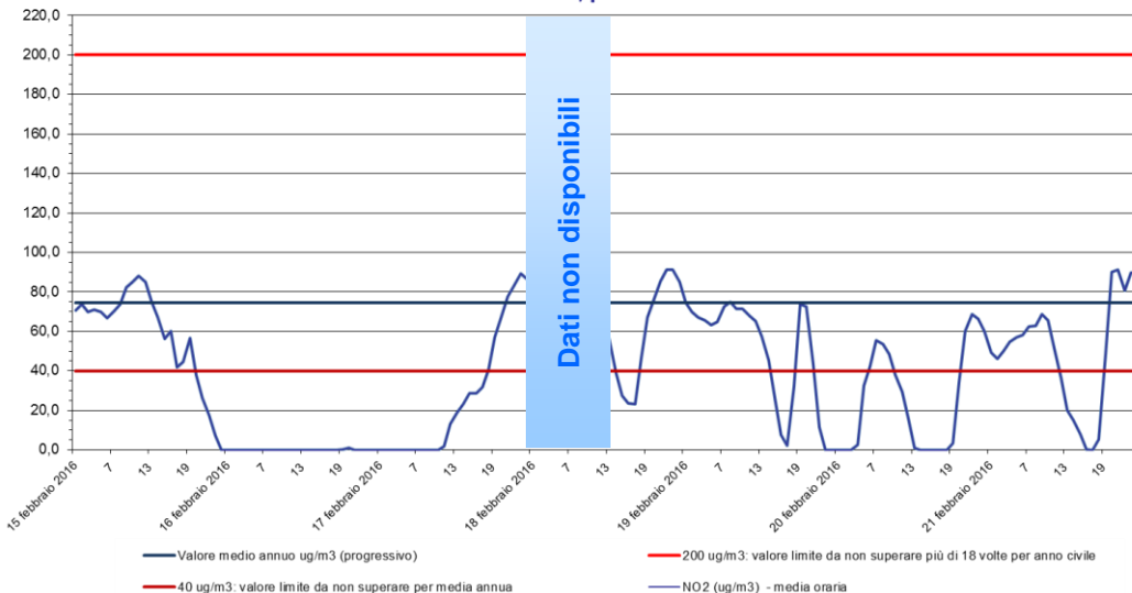
Biossido di azoto - NO 2 Stazione di rilevamento di Sambruson, periodo: 15 feb 2016 - 21 feb 2016
