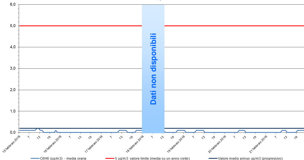
Benzene - C 6 H 6 Stazione di rilevamento di Sambruson, periodo: 15 feb 2016 - 21 feb 2016
