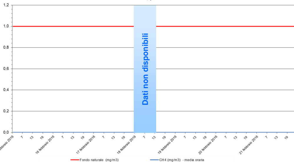
Metano - CH 4 Stazione di rilevamento di Sambruson, periodo: 15 feb 2016 - 21 feb 2016
