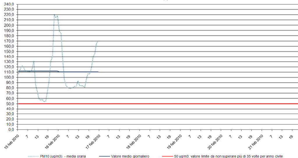
PM 10 Stazione di rilevamento di via F.lli Bandiera, periodo: 15 feb 2010 - 21 feb 2010
