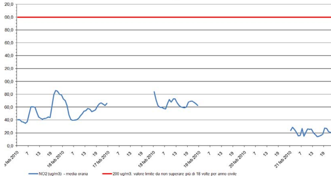
Biossido di azoto - NO 2 Stazione di rilevamento di via B. Cairoli, periodo: 15 feb 2010 - 21 feb 2010
