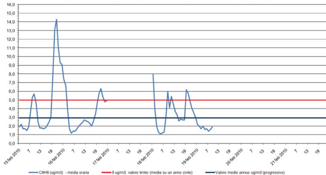
Benzene - C 6 H 6 Stazione di rilevamento di via B. Cairoli, periodo: 15 feb 2010 - 21 feb 2010
