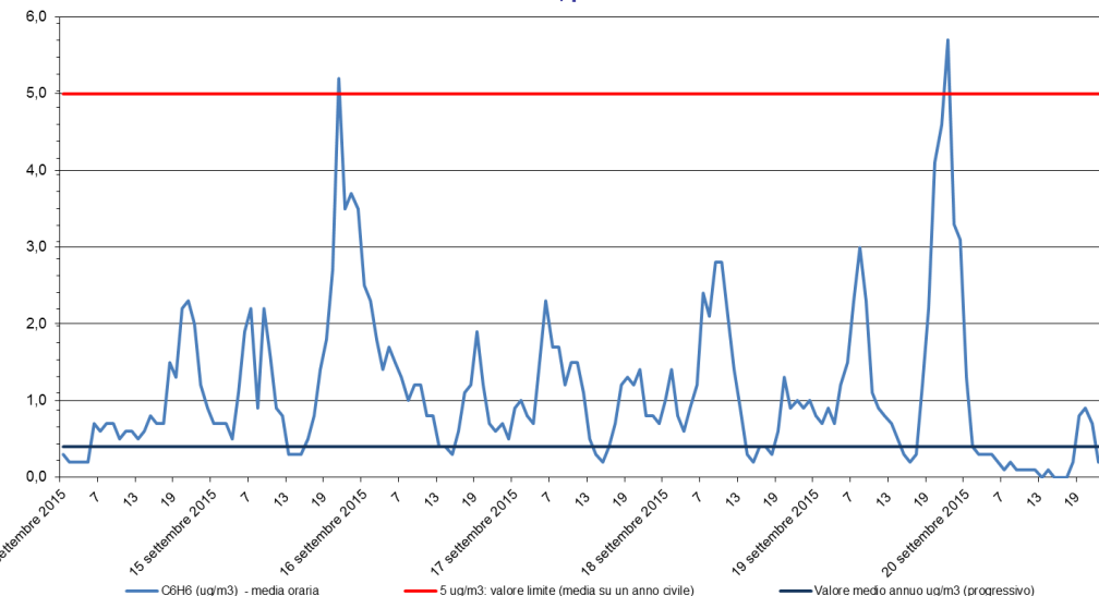
Benzene - C 6 H 6 Stazione di rilevamento di via B. Cairoli, periodo: 14 set 2015 - 20 set 2015
