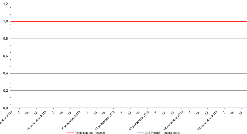
Metano - CH 4 Stazione di rilevamento di via B. Cairoli, periodo: 14 set 2015 - 20 set 2015
