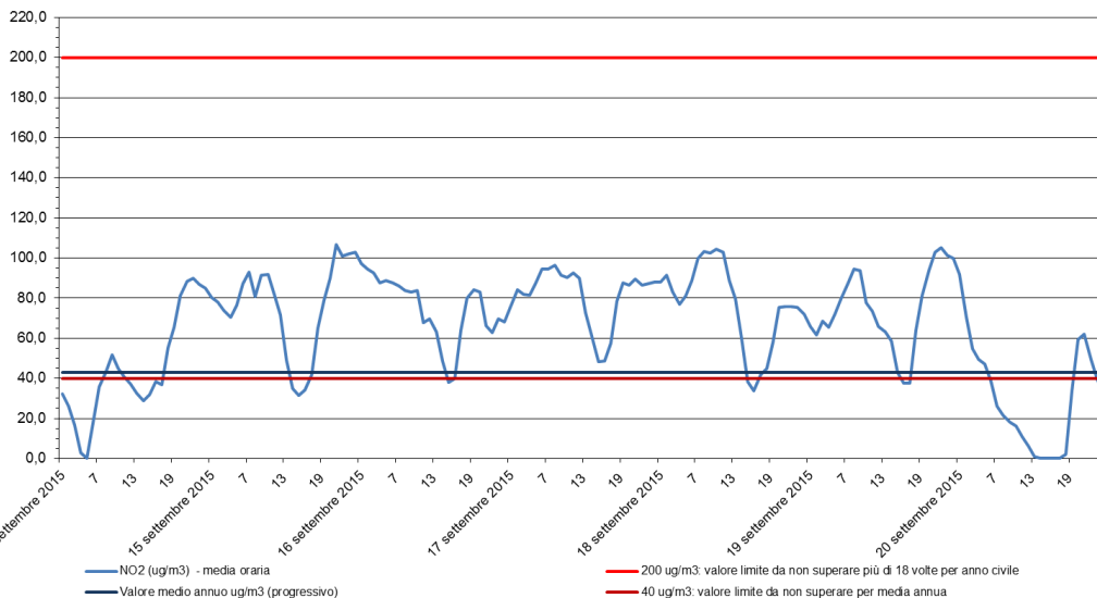
Biossido di azoto - NO 2 Stazione di rilevamento di via B. Cairoli, periodo: 14 set 2015 - 20 set 2015
