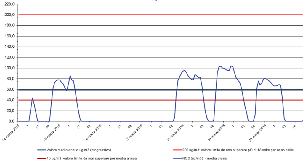
Biossido di azoto - NO 2 Stazione di rilevamento di Sambruson, periodo: 14 mar 2016 - 20 mar 2016
