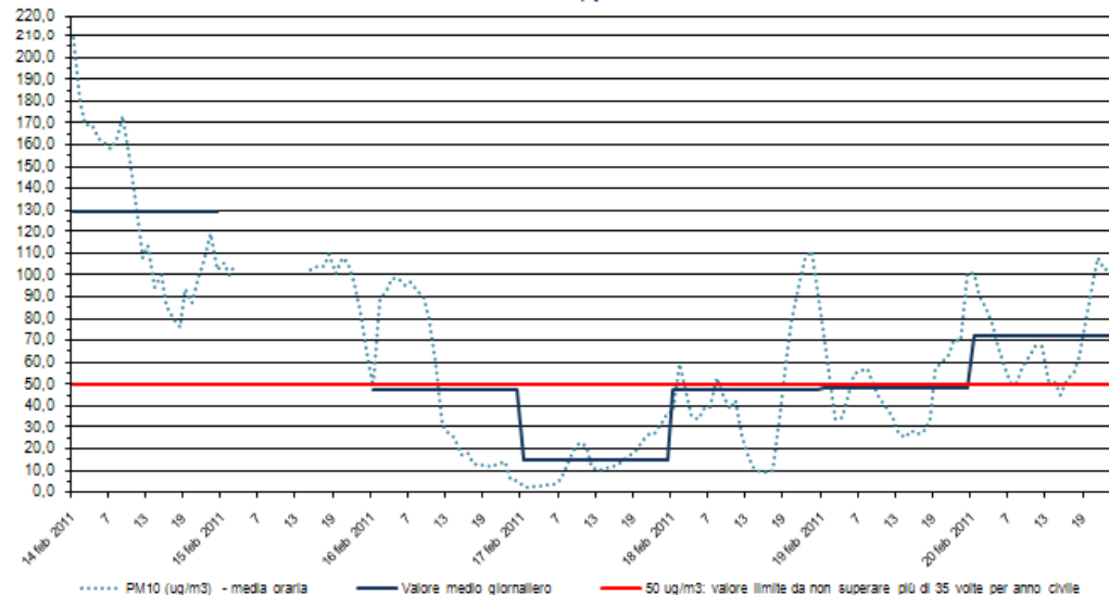
PM10 Stazione di rilevamento di via B. Cairoli, periodo: 14 feb 2011 - 20 feb 2011
