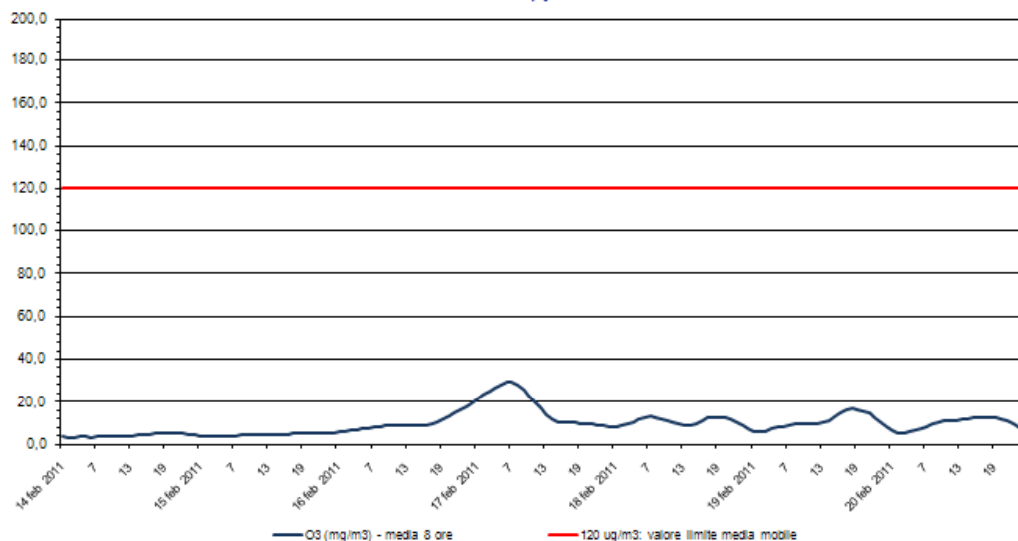
Ozono - O 3 Stazione di rilevamento di via B. Cairoli, periodo: 14 feb 2011 - 20 feb 2011
