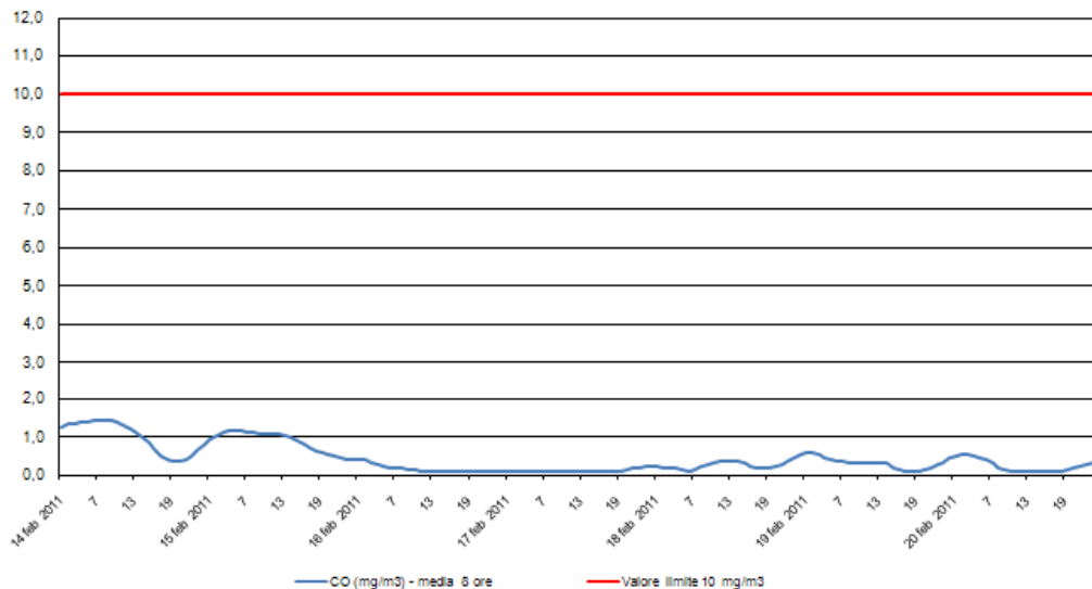
Monossido di Carbonio - CO Stazione di rilevamento di via B. Cairoli, periodo: 14 feb 2011 - 20 feb 2011
