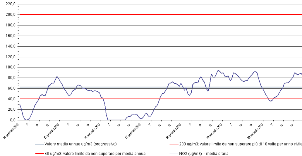
Biossido di azoto - NO 2 Stazione di rilevamento di Sambruson, periodo: 14 gen 2013 - 20 gen 2013
