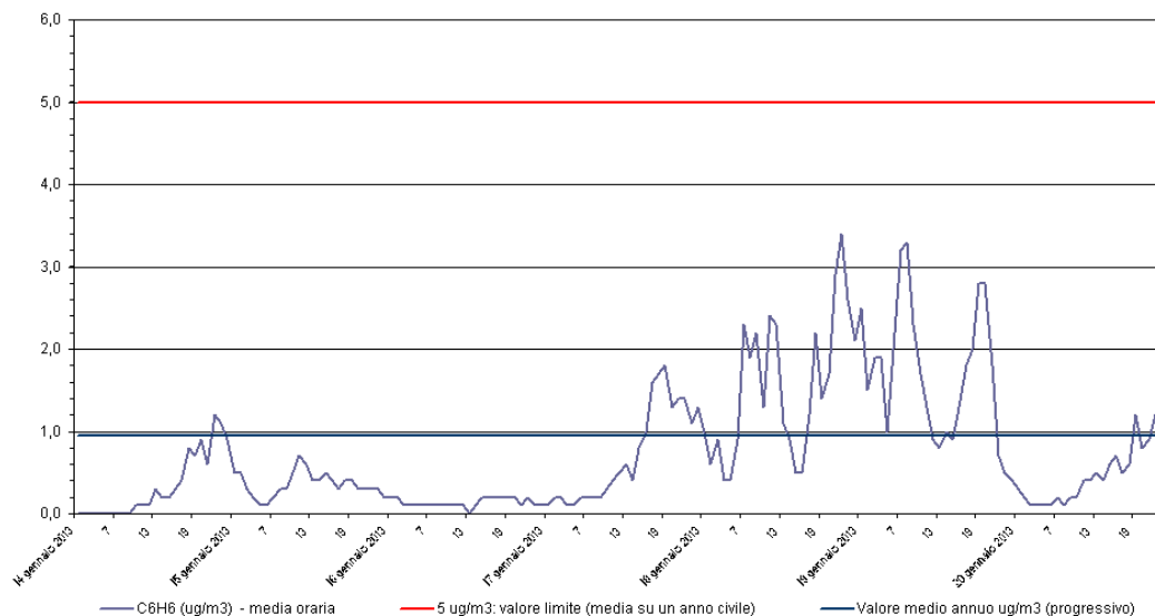
Benzene - C 6 H 6 Stazione di rilevamento di Sambruson, periodo: 14 gen 2013 - 20 gen 2013
