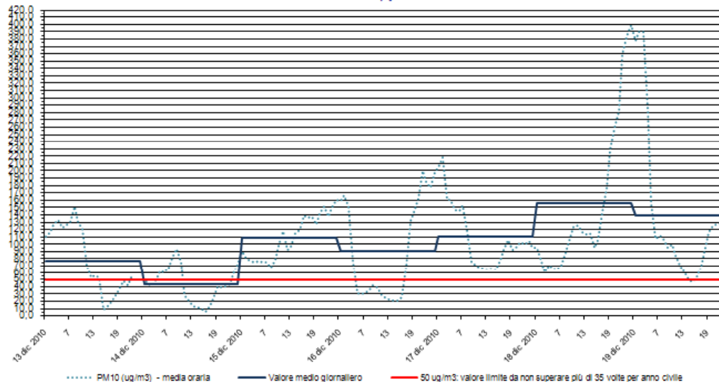
PM 10 Stazione di rilevamento di via B. Cairoli, periodo: 13 dic 2010 - 19 dic 2010
