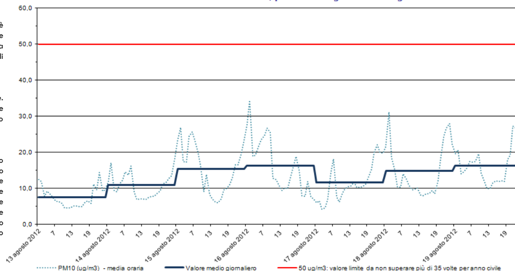
PM 10 Stazione di rilevamento di via B. Cairoli, periodo: 13 ago 2012 - 19 ago 2012
