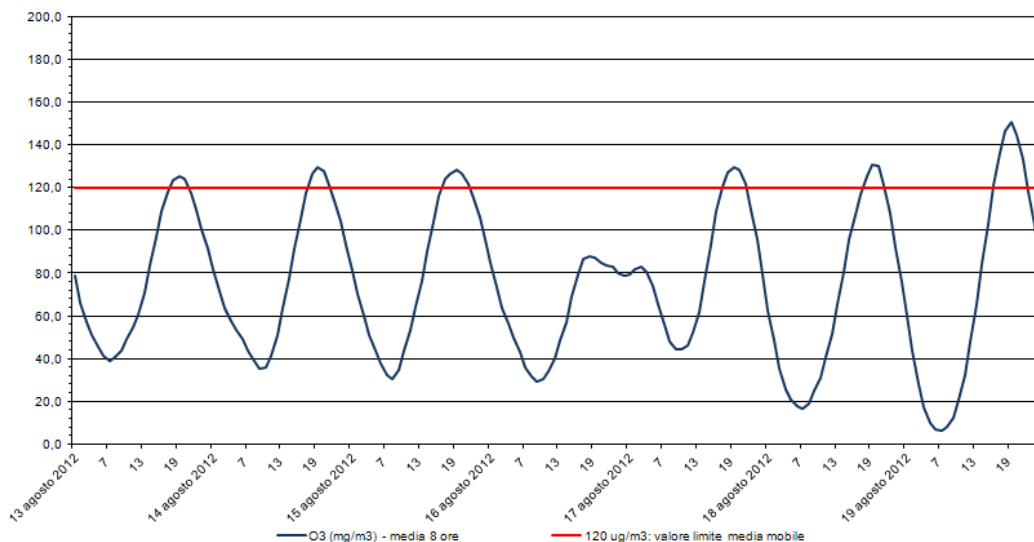
Ozono - O3 Stazione di rilevamento di via B. Cairoli, periodo: 13 ago 2012 - 19 ago 2012
