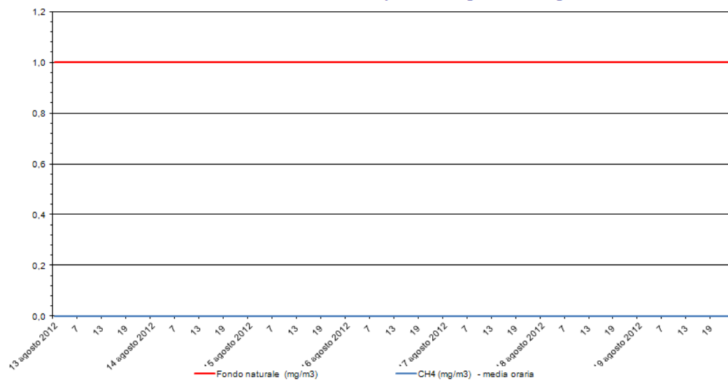
Metano - CH 4 Stazione di rilevamento di via B. Cairoli, periodo: 13 ago 2012 - 19 ago 2012
