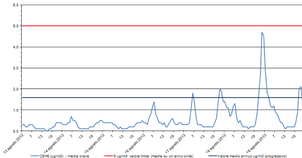
Benzene - C 6 H 6 Stazione di rilevamento di via B. Cairoli, periodo: 13 ago 2012 - 19 ago 2012
