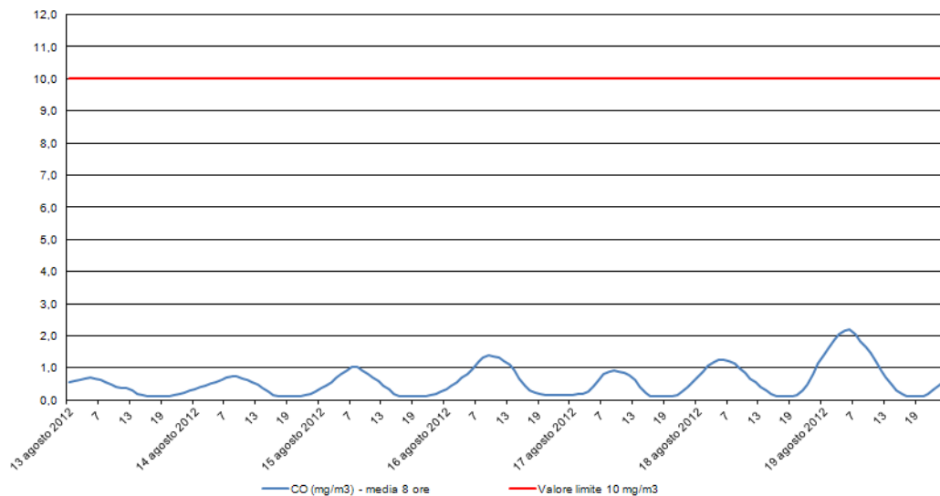
Monossido di Carbonio - CO Stazione di rilevamento di via B. Cairoli, periodo: 13 ago 2012 - 19 ago 2012
