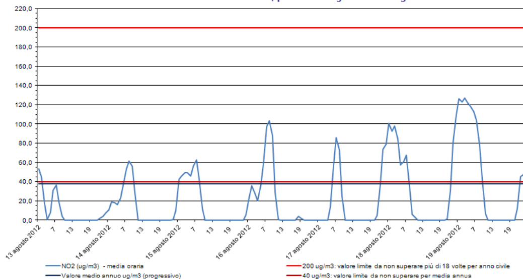
Biossido di azoto - NO 2 Stazione di rilevamento di via B. Cairoli, periodo: 13 ago 2012 - 19 ago 2012
