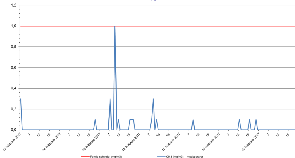
Metano - CH 4 Stazione di rilevamento di Sambruson, periodo: 13 feb 2017 - 19 feb 2017
