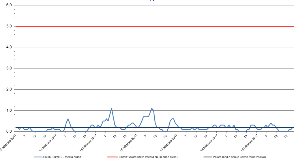
Benzene - C 6 H 6 Stazione di rilevamento di Sambruson, periodo: 13 feb 2017 - 19 feb 2017
