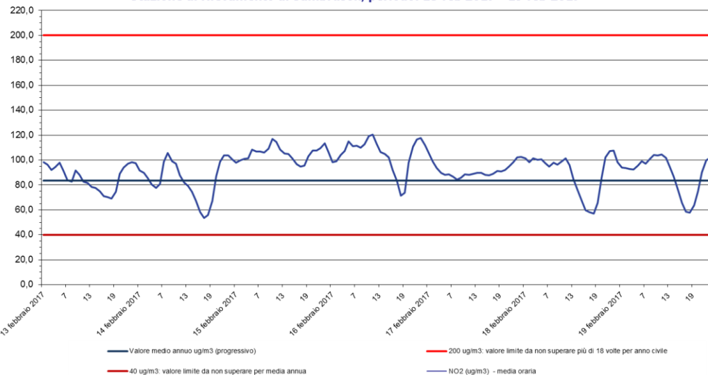
Biossido di azoto - NO 2 Stazione di rilevamento di Sambruson, periodo: 13 feb 2017 - 19 feb 2017
