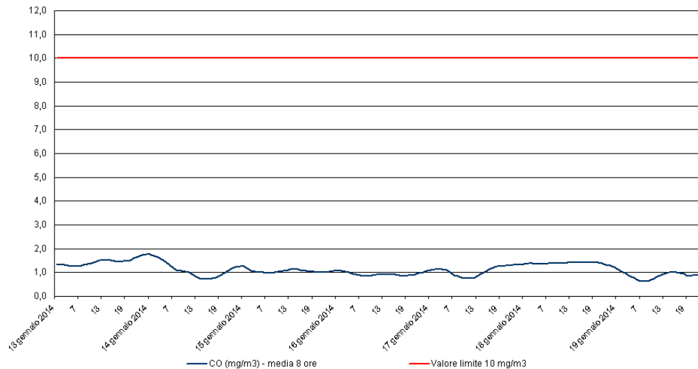
Monossido di Carbonio - CO Stazione di rilevamento di Sambruson, periodo: 13 gen 2014 - 19 gen 2014
