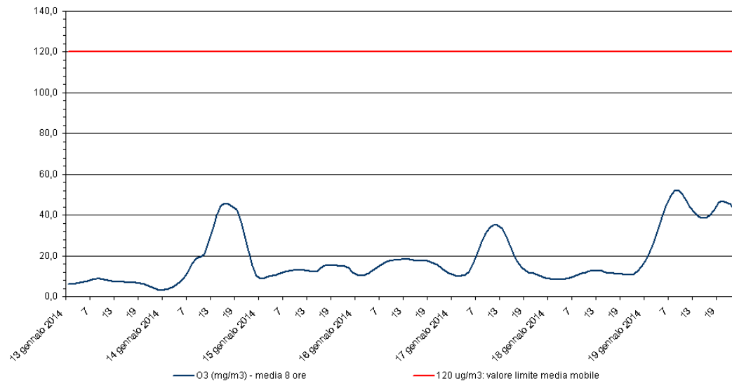
Ozono - O 3 Stazione di rilevamento di Sambruson, periodo: 13 gen 2014 - 19 gen 2014
