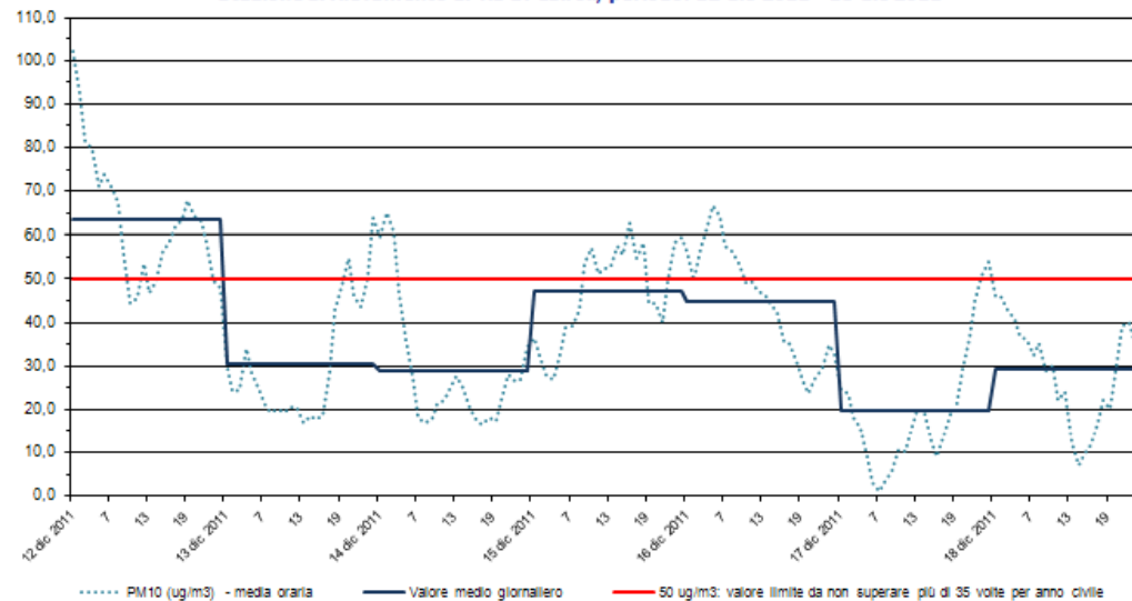
PM10 Stazione di rilevamento di via B. Cairoli, periodo: 12 dic 2011 - 18 dic 2011
