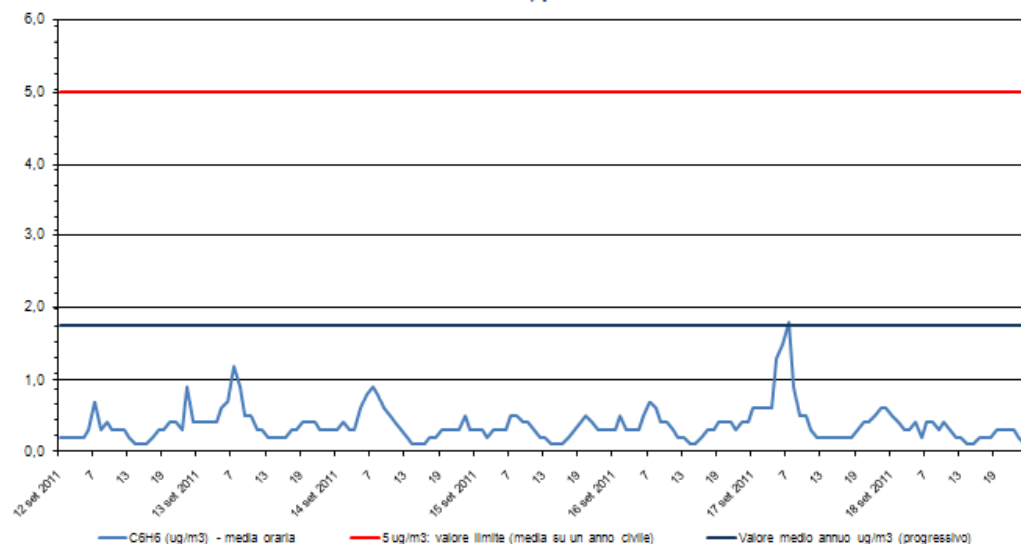
Benzene - C 6 H 6 Stazione di rilevamento di via B. Cairoli, periodo: 12 set 2011 - 18 set 2011
