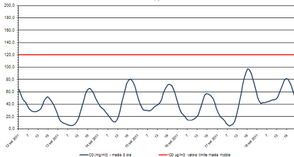
Ozono - O 3 Stazione di rilevamento di via B. Cairoli, periodo: 12 set 2011 - 18 set 2011
