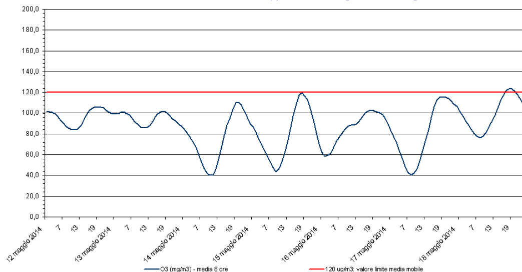
Ozono - O 3 Stazione di rilevamento di via B. Cairoli, periodo: 12 mag 2014 - 18 mag 2014
