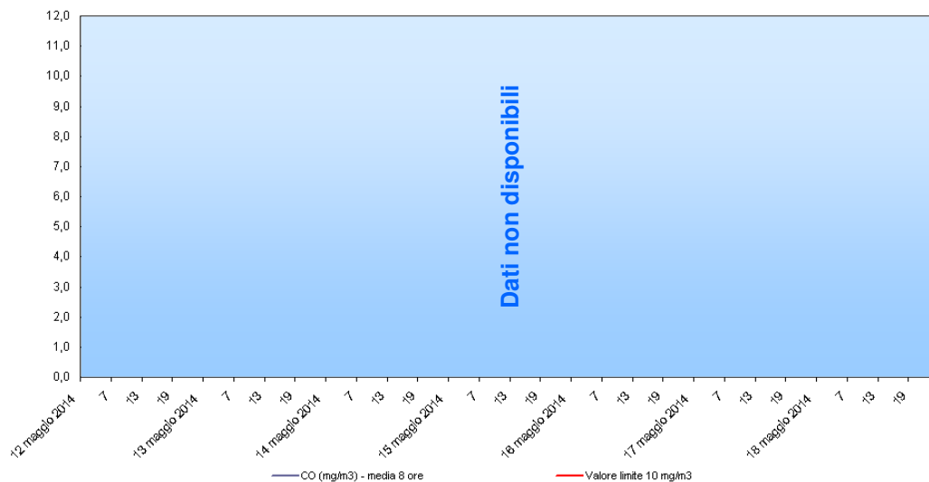
Monossido di Carbonio - CO Stazione di rilevamento di via B. Cairoli, periodo: 12 mag 2014 - 18 mag 2014
