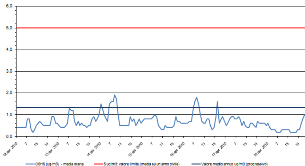
Benzene - C 6 H 6 Stazione di rilevamento di via F.lli Bandiera, periodo: 12 apr 2010 - 18 apr 2010
