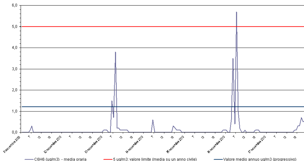
Benzene - C 6 H 6 Stazione di rilevamento di Sambruson, periodo: 11 nov 2013 - 17 nov 2013
