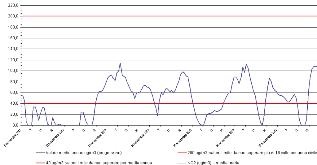
Biossido di azoto - NO 2 Stazione di rilevamento di Sambruson, periodo: 11 nov 2013 - 17 nov 2013
