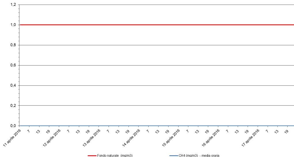
Metano - CH 4 Stazione di rilevamento di via B. Cairolì, periodo: 11 apr 2016 - 17 apr 2016
