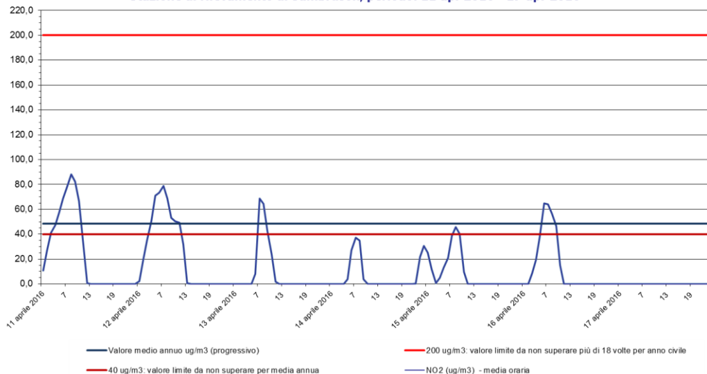
Biossido di azoto - NO 2 Stazione di rilevamento di Sambruson, periodo: 11 apr 2016 - 17 apr 2016
