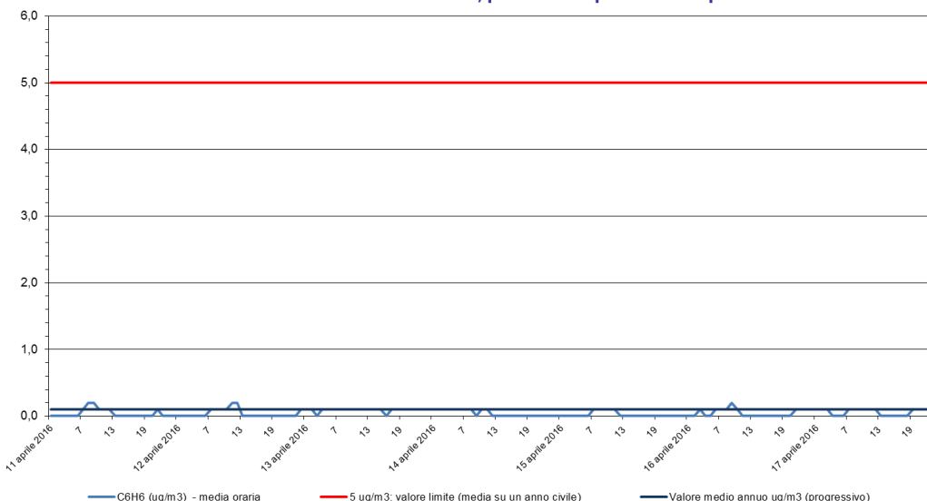
Benzene - C 6 H 6 Stazione di rilevamento di Sambruson, periodo: 11 apr 2016 - 17 apr 2016
