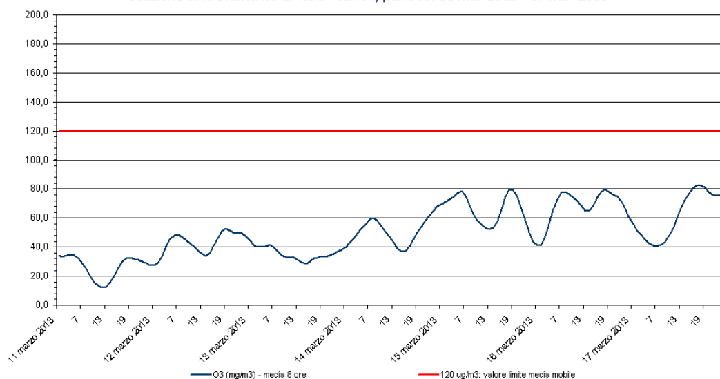
Ozono - O 3 Stazione di rilevamento di via B. Cairoli, periodo: 11 mar 2013 - 17 mar 2013
