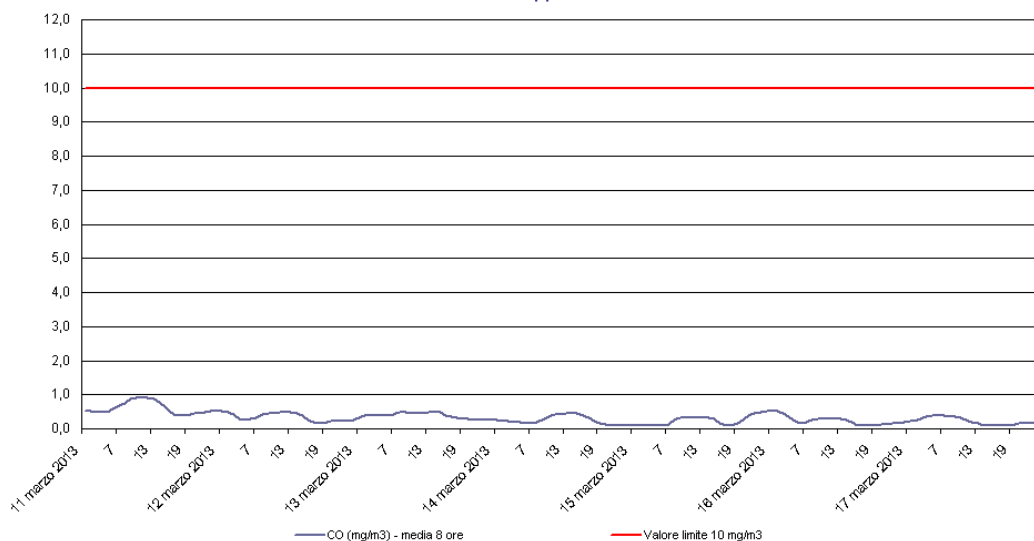
Monossido di Carbonio - CO Stazione di rilevamento di via B. Cairoli, periodo: 11 mar 2013 - 17 mar 2013
