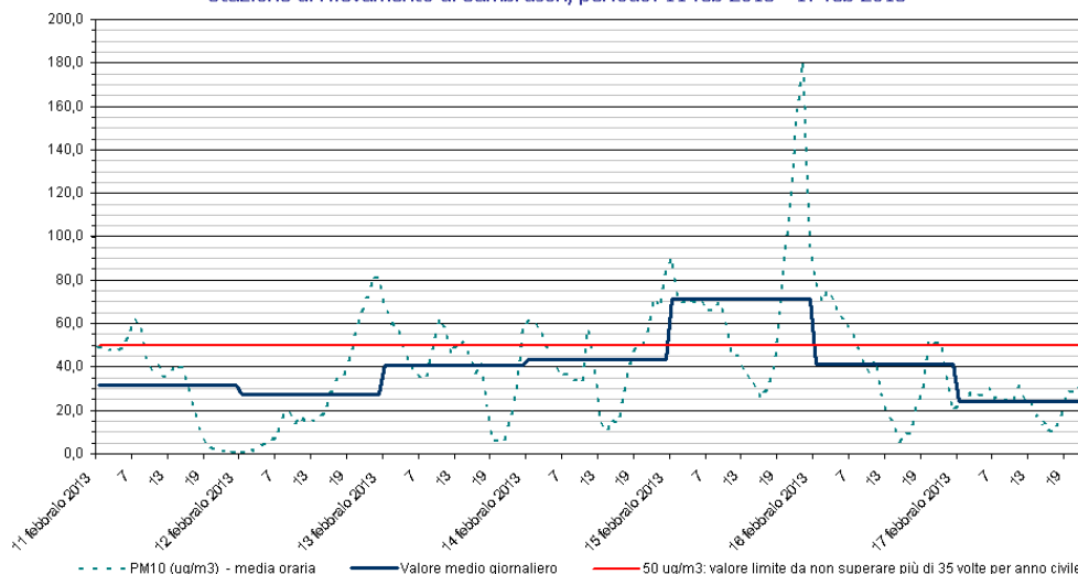
PM10 Stazione di rilevamento di Sambruson, periodo: 11 feb 2013 - 17 feb 2013
