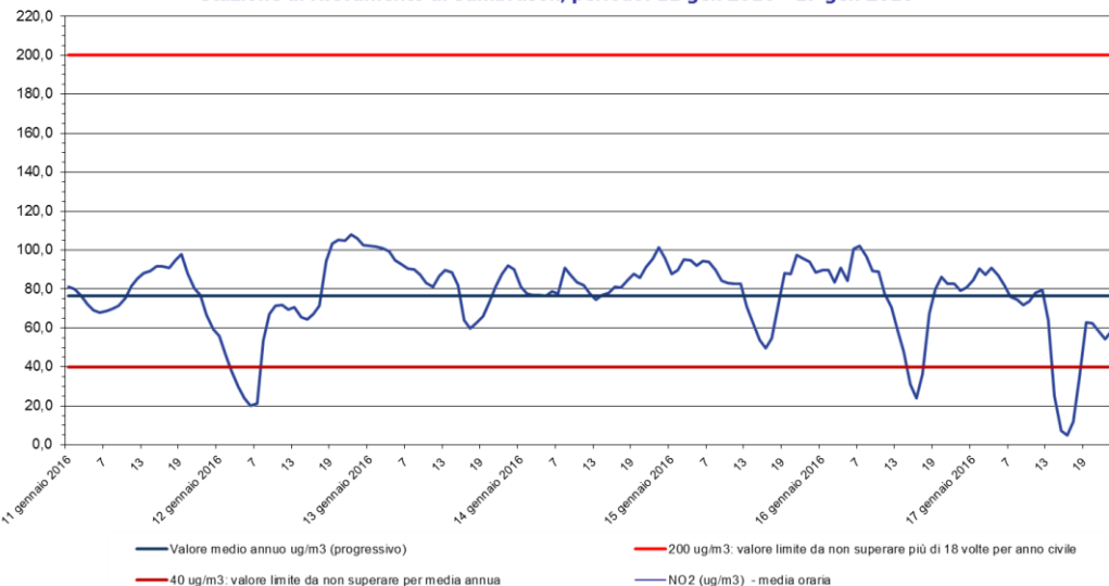
Biossido di azoto - NO 2 Stazione di rilevamento di Sambruson, periodo: 11 gen 2016 - 17 gen 2016
