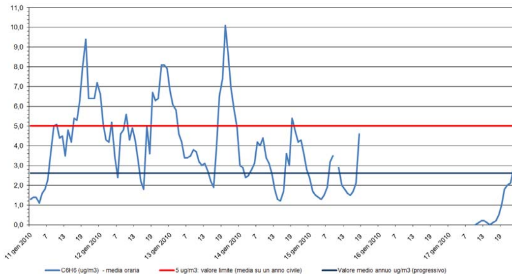
Benzene - C 6 H 6 Stazione di rilevamento di via B. Cairoli, periodo: 11 gen 2010 - 17 gen 2010
