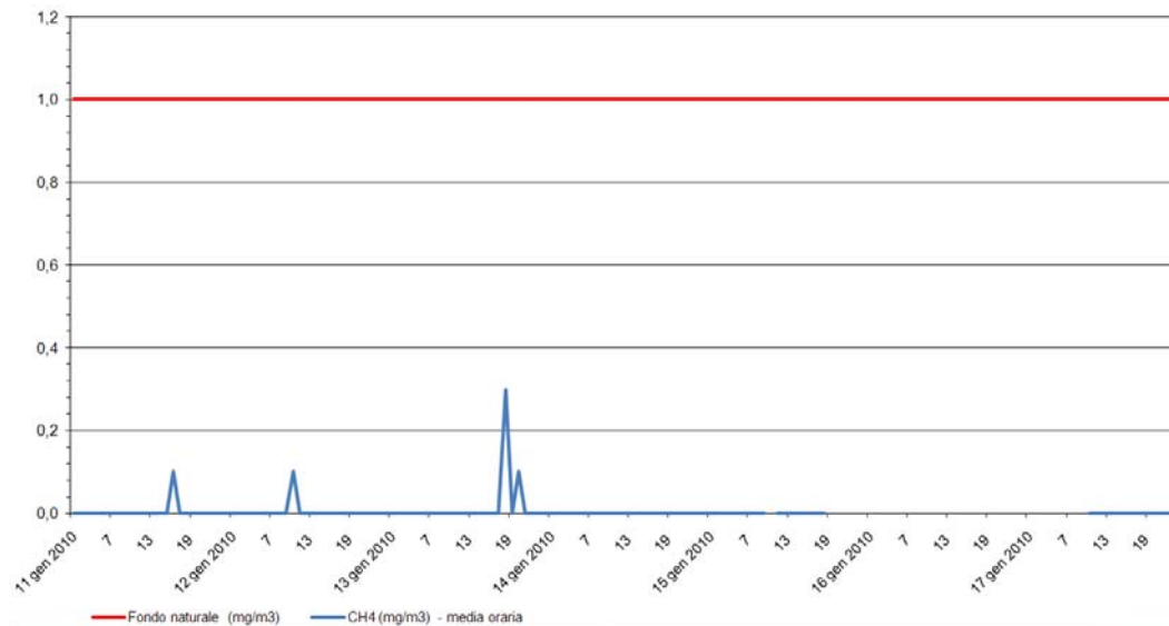
Metano - CH 4 Stazione di rilevamento di via B. Cairoli, periodo: 11 gen 2010 - 17 gen 2010
