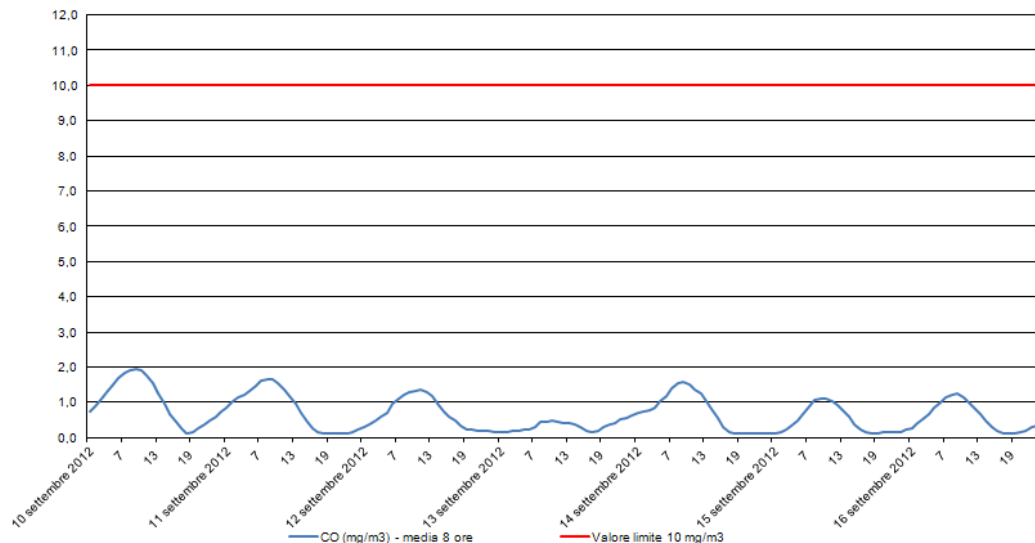
Monossido di Carbonio - CO Stazione di rilevamento di via B. Cairoli, periodo: 10 set 2012 - 16 set 2012
