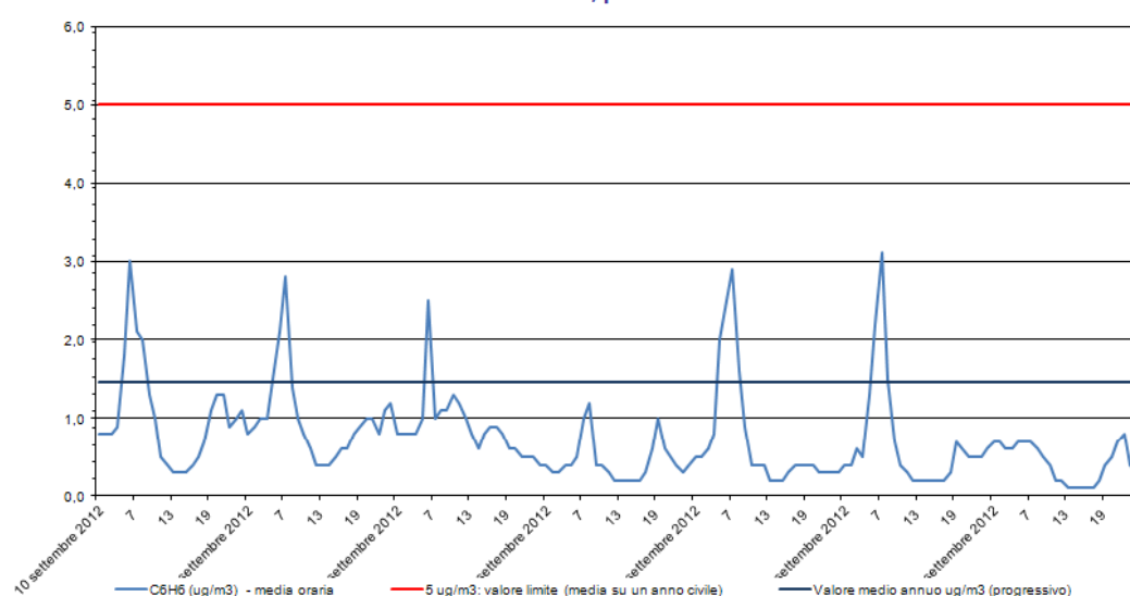
Benzene - C 6 H 6 Stazione di rilevamento di via B. Cairoli, periodo: 10 set 2012 - 16 set 2012
