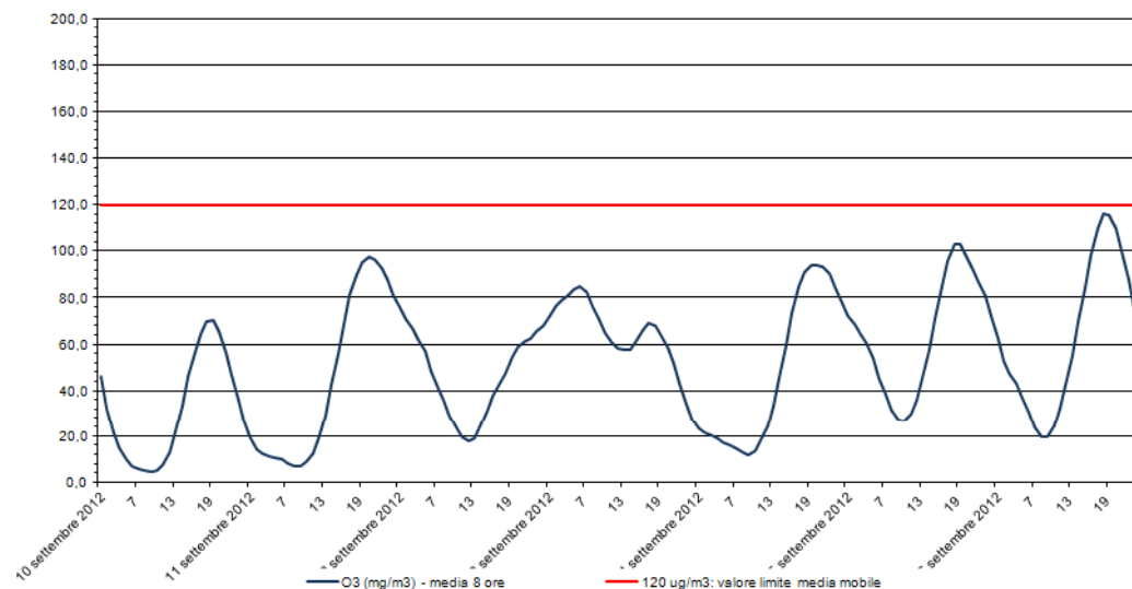
Ozono - O3 Stazione di rilevamento di via B. Cairoli, periodo: 10 set 2012 - 16 set 2012
