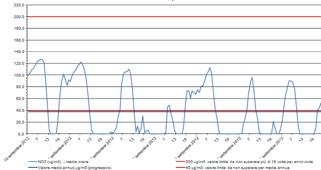
Biossido di azoto - NO 2 Stazione di rilevamento di via B. Cairoli, periodo: 10 set 2012 - 16 set 2012
