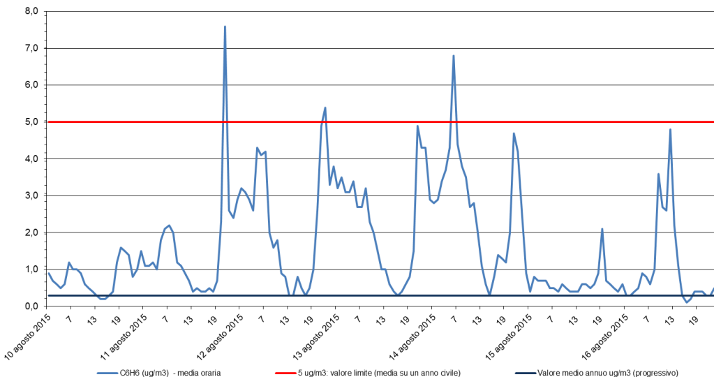
Benzene - C 6 H 6 Stazione di rilevamento di via B. Cairoli, periodo: 10 ago 2015 - 16 ago 2015
