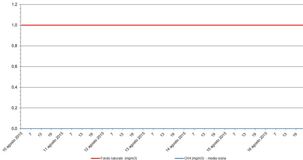
Metano - CH 4 Stazione di rilevamento di via B. Cairoli, periodo: 10 ago 2015 - 16 ago 2015
