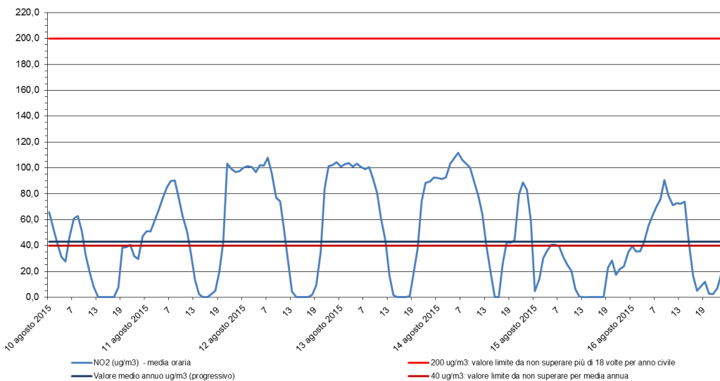
Biossido di azoto - NO 2 Stazione di rilevamento di via B. Cairoli, periodo: 10 ago 2015 - 16 ago 2015
