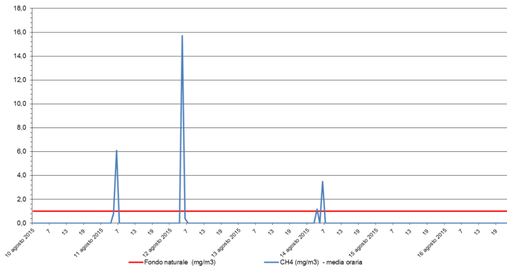
Metano - CH 4 Stazione di rilevamento di Sambruson, periodo: 10 ago 2015 - 16 ago 2015
