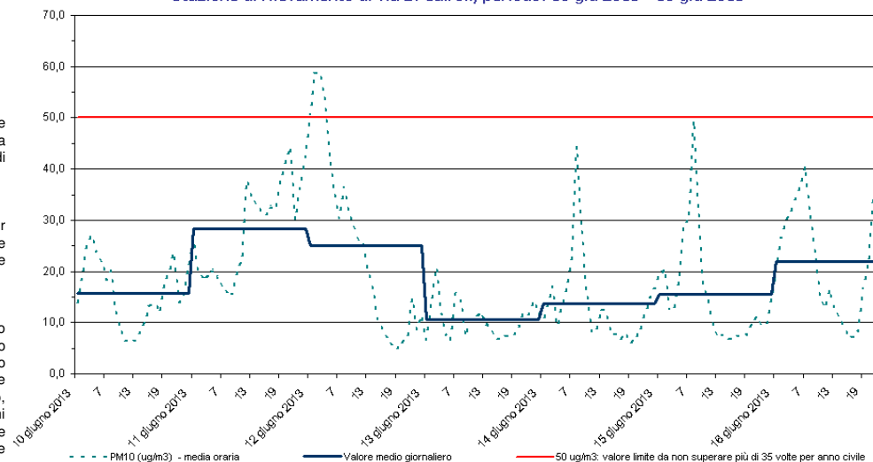
PM10 Stazione di rilevamento di via B. Cairoli, periodo: 10 giu 2013 - 16 giu 2013
