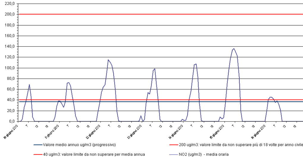
Biossido di azoto - NO 2 Stazione di rilevamento di Sambruson, periodo: 10 giu 2013 - 16 giu 2013
