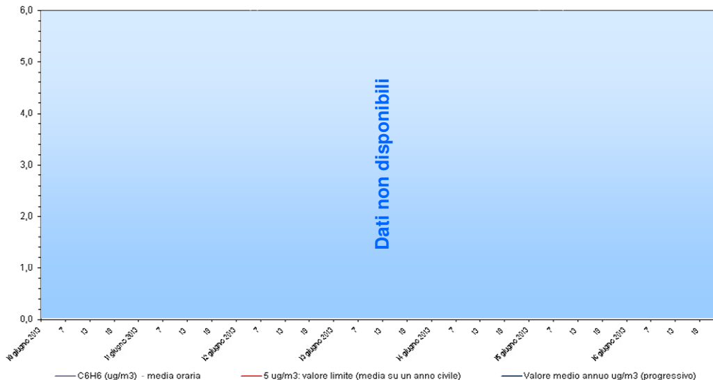
Benzene - C 6 H 6 Stazione di rilevamento di Sambruson, periodo: 10 giu 2013 - 16 giu 2013
