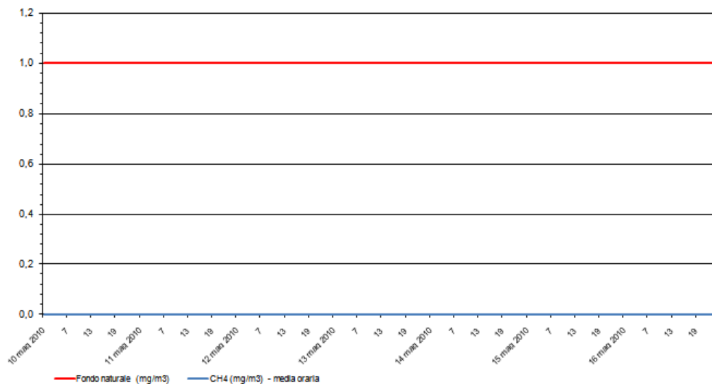
Metano - CH 4 Stazione di rilevamento di via F.lli Bandiera, periodo: 10 mag 2010 - 16 mag 2010
